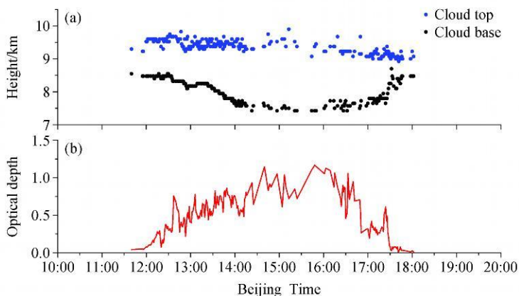
图 5 2007 年 6 月 1 日 10:00~20:00 (a) 卷云高度和 (b) 光学厚度随时间变化
