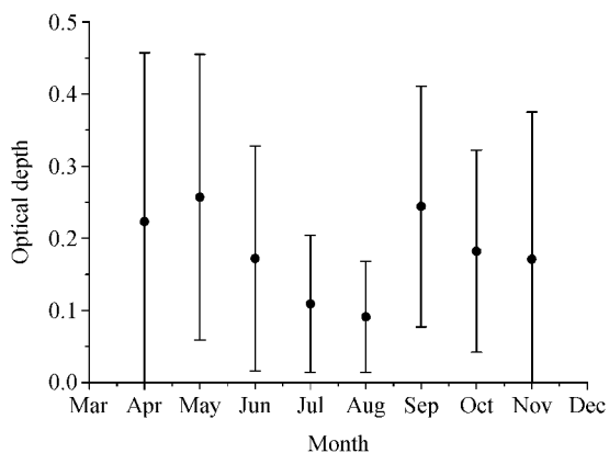
图10 卷云光学厚度月变化特征
