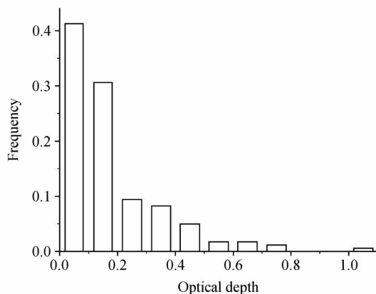
图9 卷云光学厚度频数分布
