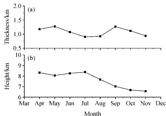
图8 (a) 卷云厚度和 (b) 云底高度月变化特征
