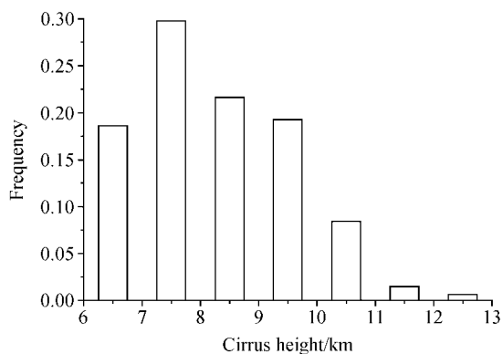
图 6 卷云高度频数分布
