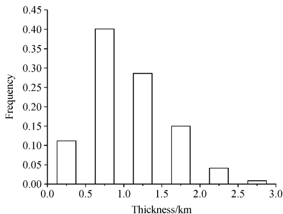
图7 卷云厚度频数分布
