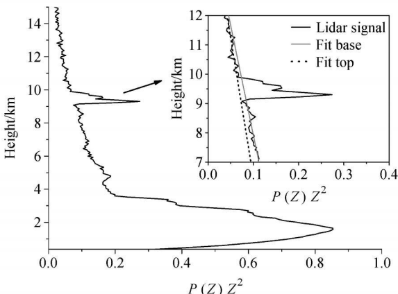
图3 透过率法求解卷云光学厚度示意图
