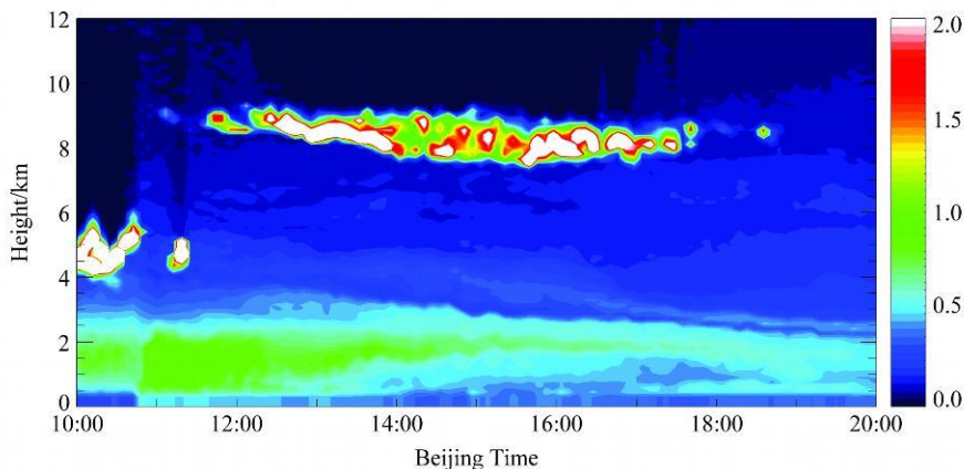
图 4 2007 年 6 月 1 日 10:00~20:00 卷云雷达信号强度时空分布特征
