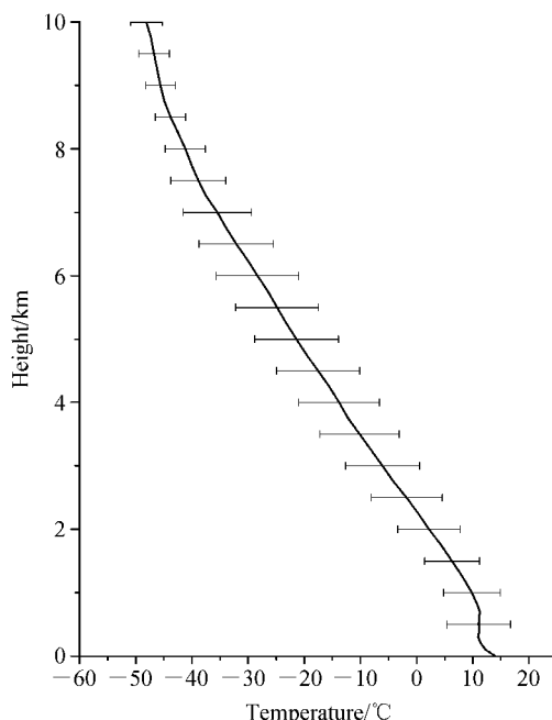
图 1 SACOL 年平均温度垂直分布
