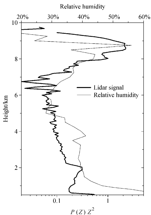
图 2 2007 年 9 月 8 日 11: 26 (北京时, 下同) 雷达回波信号及水汽垂直分布
