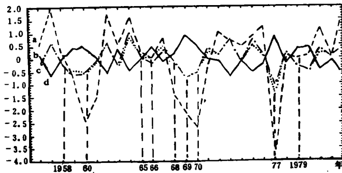
图 2e 各层第一特征向量的时间系数演变 (a, 100hPa(虚线), b, 500hPa(点划线), c, 700hPa(点线), d, 1000hPa(实线))
