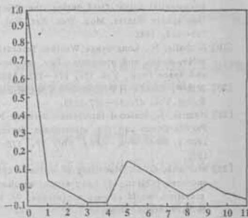
图 3a(左)起始月为 1 月的回归直线的斜率变化
