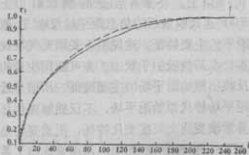
图 2 相关系数( r_i )随信息点数( i )增加的演变曲线。实线为冬季 1 月, 虚线为夏季 7 月
